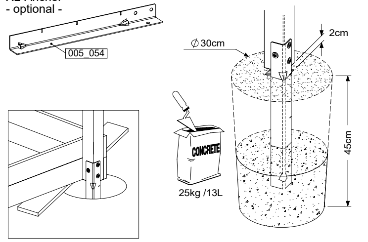
XL-Anchor - optional -
